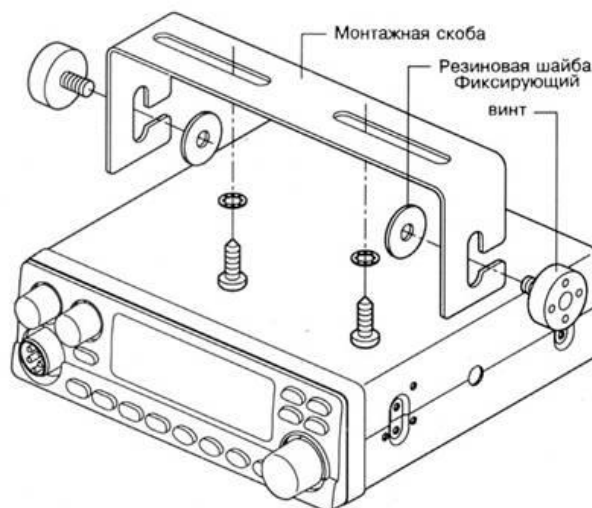
Рис.1. Крепление радиостанции при помощи монтажной скобы.
